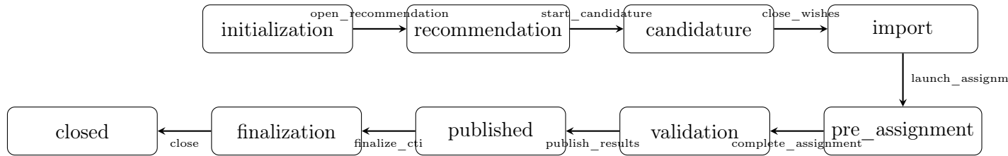
FIGURE 4.1 – Machine à états : AcademicYear
