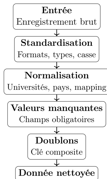
FIGURE 3.4 – Pipeline détaillé de l'étape de nettoyage des données
