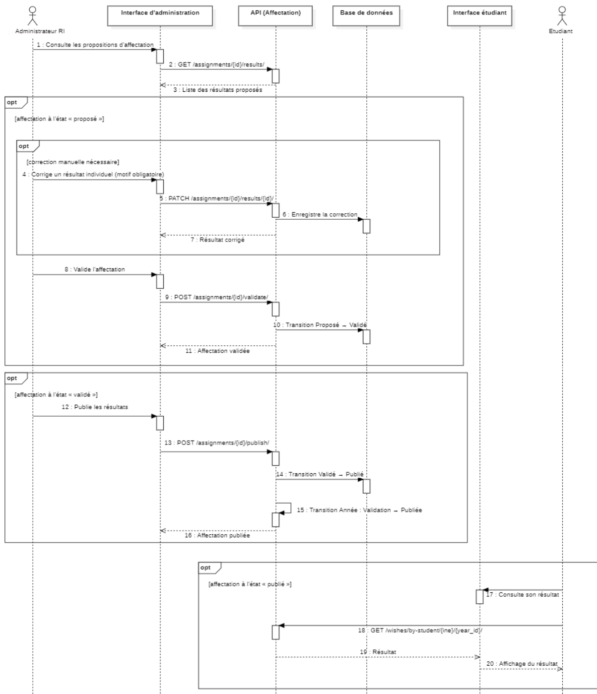
FIGURE 5.11 – Diagramme de séquence : validation, correction et publication des affectations
