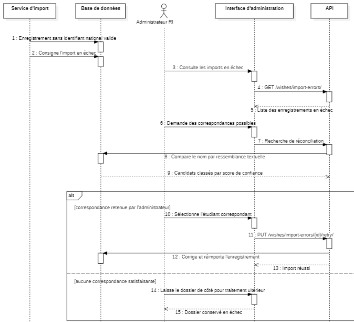
FIGURE 5.15 – Diagramme de séquence : réconciliation d'un dossier sans identifiant valide
