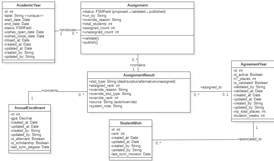
FIGURE 5.9 – Diagramme de classes : Sprint 3
