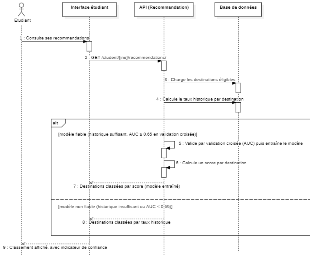
FIGURE 5.22 – Diagramme de séquence : calcul et consultation d'une recommandation de destination
