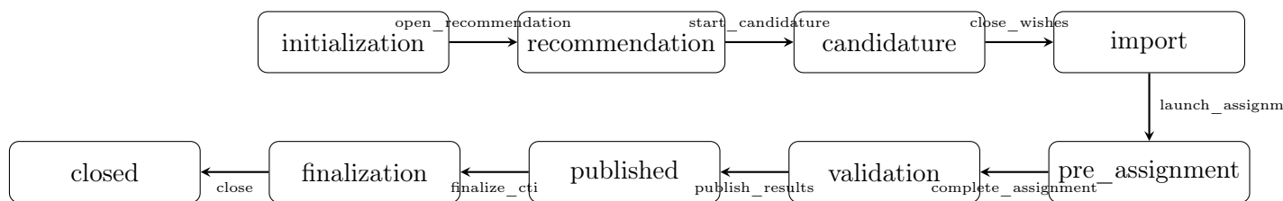
FIGURE 3.3 – Machine à états — AcademicYear
