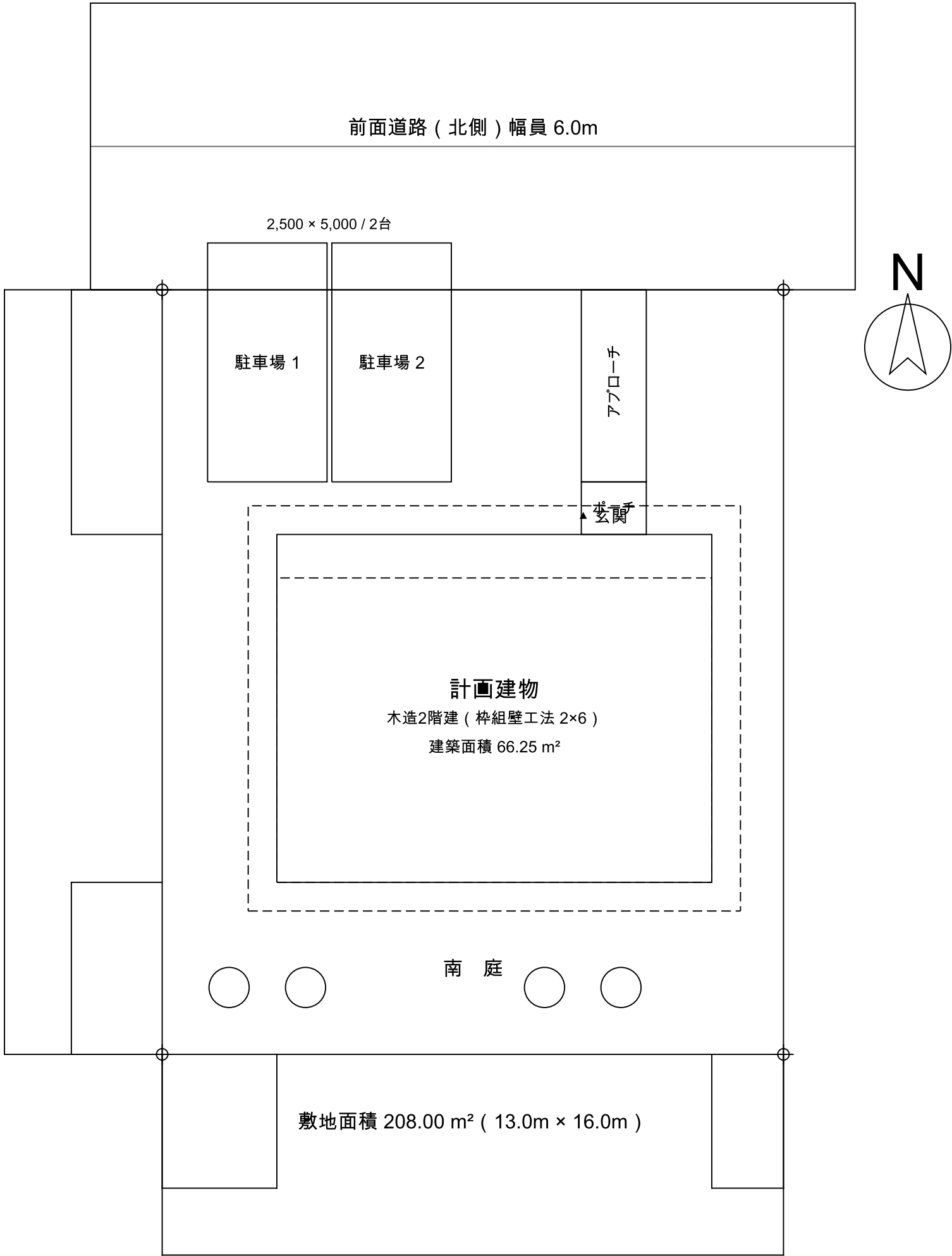
配 置 図 S=1:100
