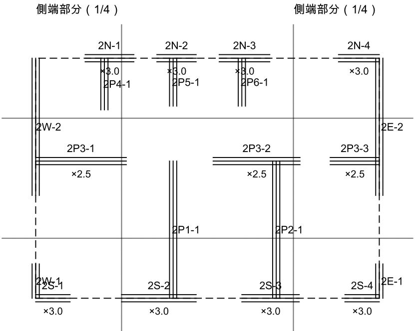
2階 耐力壁配置図 S=1:100
