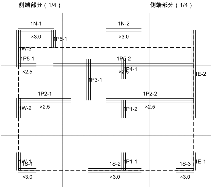
1階 耐力壁配置図 S=1:100
