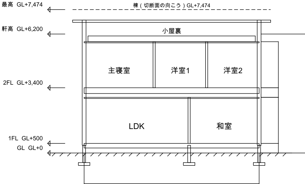
B-B' 断面図 S=1:100
