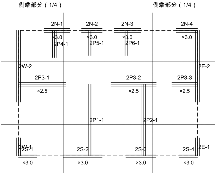
2階 耐力壁配置図 S=1:100
