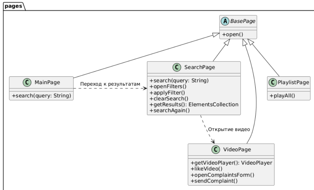
Рисунок 22 – Диаграмма классов страниц (Пакет pages)
