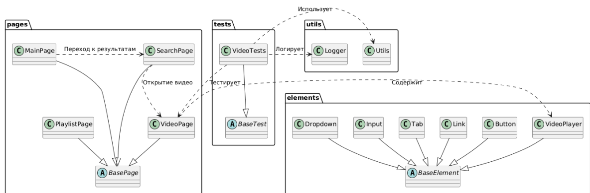
Рисунок 24 – Общая UML-диаграмма
