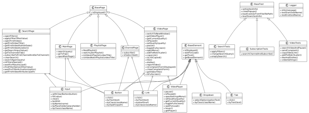
Рисунок 21 – UML-диаграмма проекта
