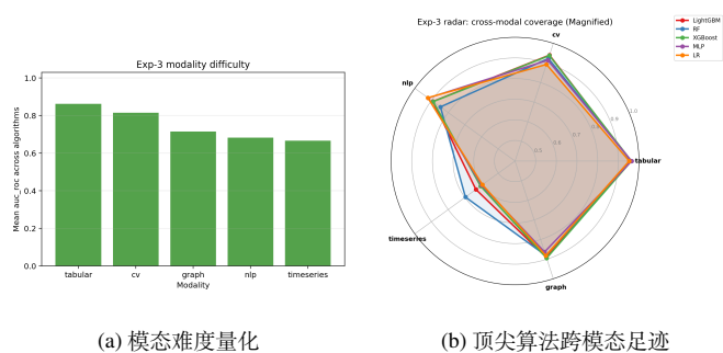
图 9 Exp3 跨模态难度与顶尖算法的多模态性能足迹
