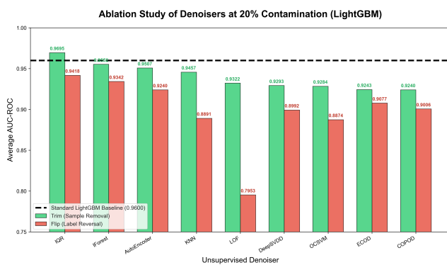
图 11 Exp4 不同清洁剂与策略 (Trim/Flip) 的去噪性能提升消融
