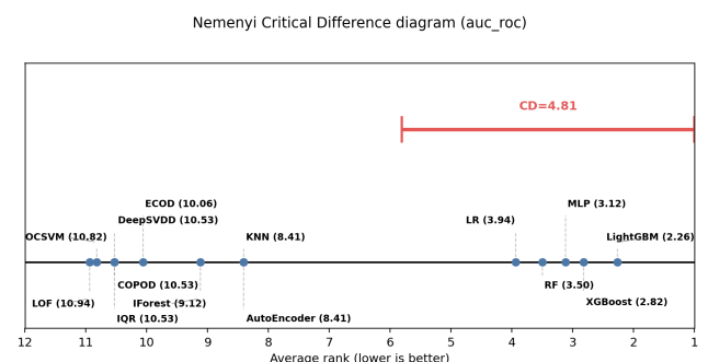
图 4 Exp1 Nemenyi 关键差值 (CD) 图：横轴为 Friedman 平均秩，横线相连者差异不显著
