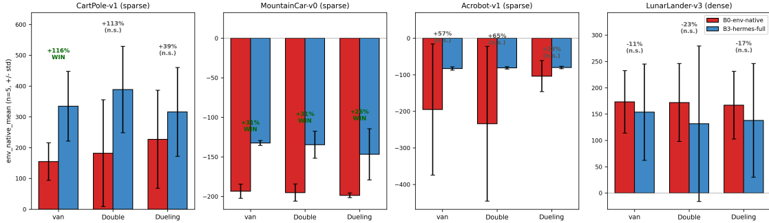
圖 4. Part 2 主結果: 三種 DQN 變體、四個環境下之 B3-hermes-full 對 B0-env-native。MountainCar 在三種變體下皆呈現 Hermes 勝出; LunarLander 在任一變體下皆未勝出。
