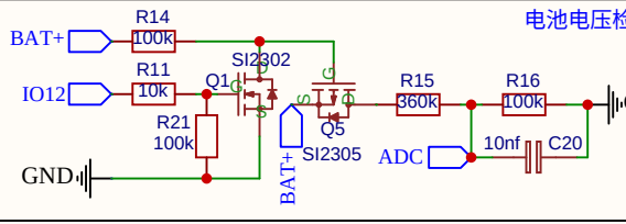
电池电压检测
