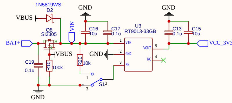
LDO与供电切换
