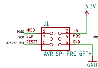
AVR ISCP
