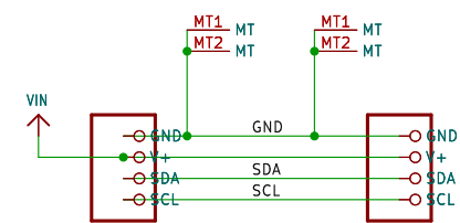
STEMMA/I2C Headers
