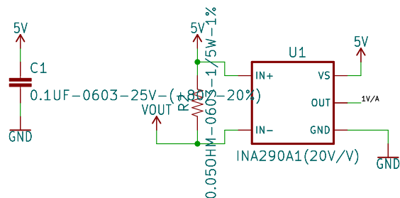
INA290
