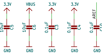
DECOUPLING CAPS
