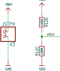
JST PH LIPO INPUT
