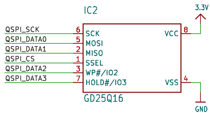
16MBIT QSPI FLASH
