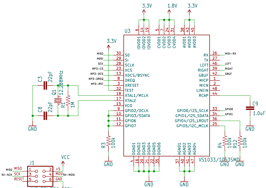
VS1053
