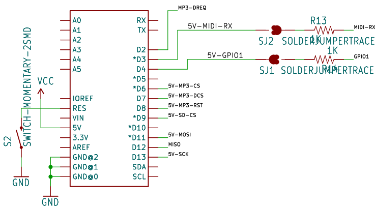
Arduino
