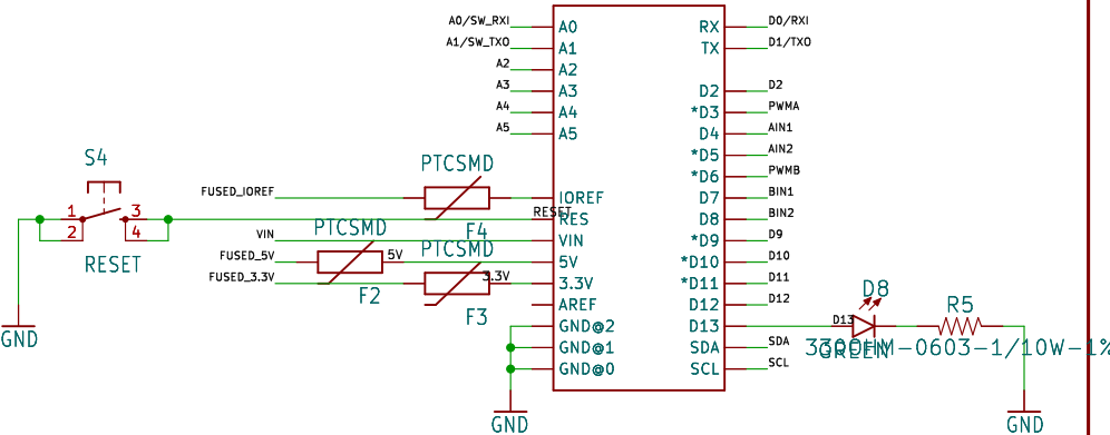
Arduino Shield
