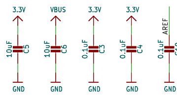
DECOUPLING CAPS
