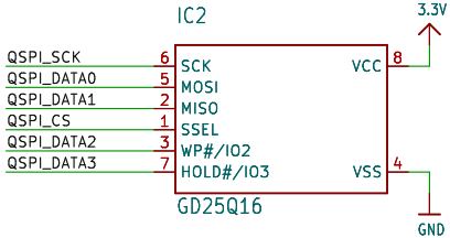
16MBIT QSPI FLASH
