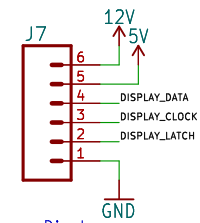
Display
