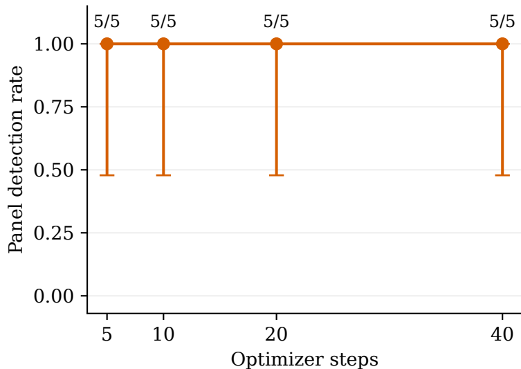
LoRA fine-tuning
