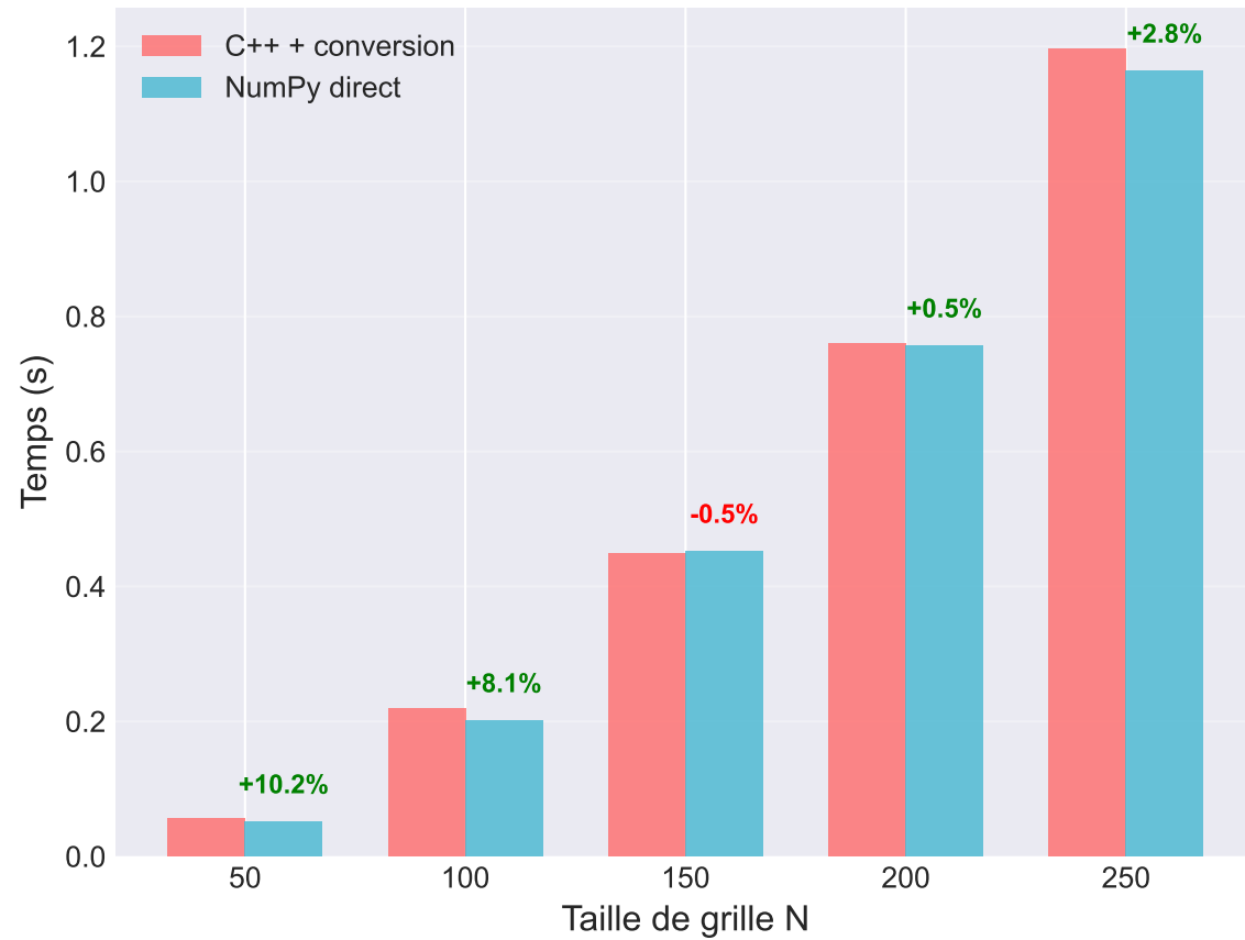
Comparaison directe des temps d'exécution
