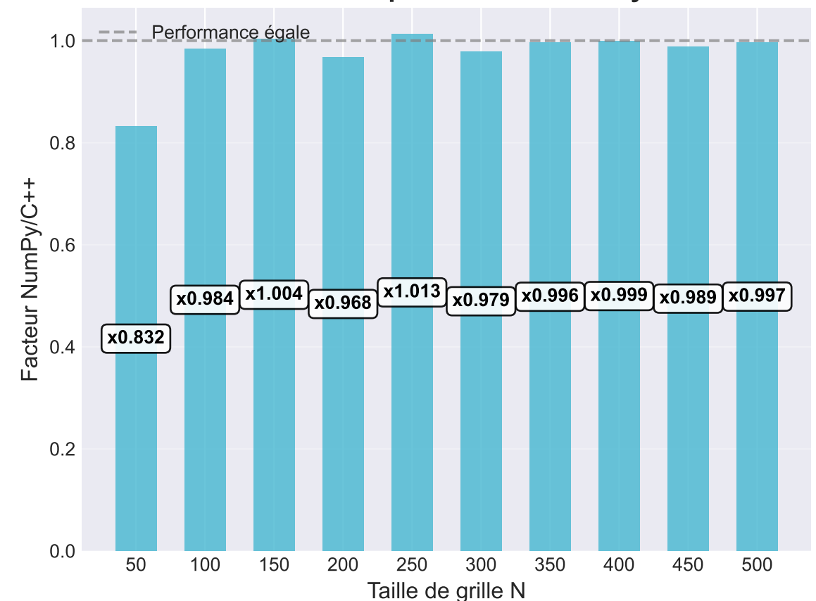
Facteur de performance NumPy
