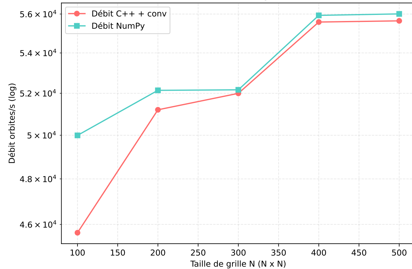
Débit orbites/s (log scale)
