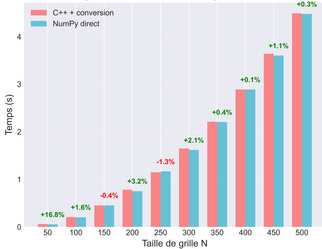
Comparaison directe des temps d'exécution
