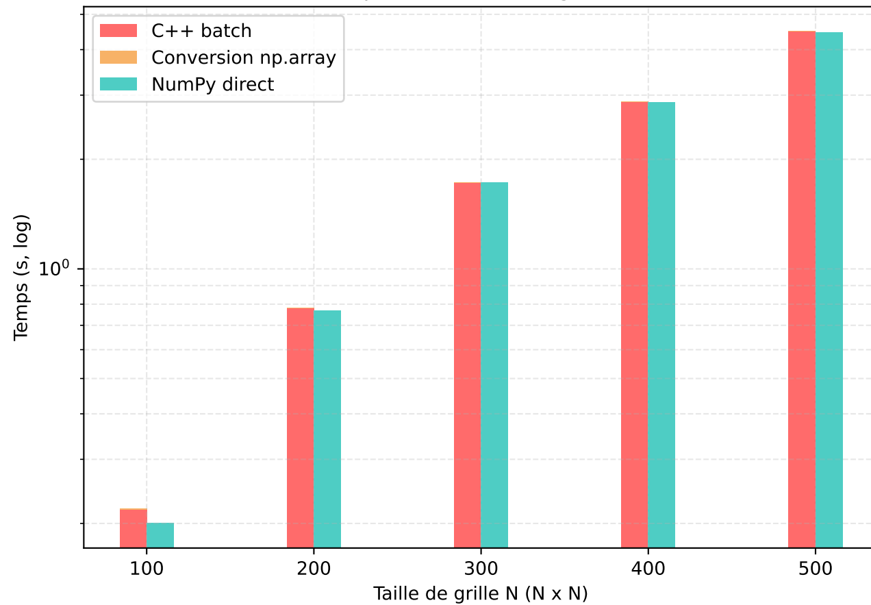
Temps d'exécution (log scale)
