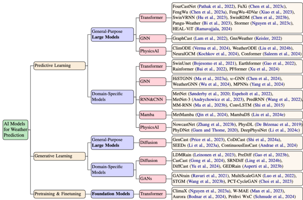
3. ábra. Az MLWP-modellek áttekintése. Az ábra Shi et al. (2025) [26] cikkéből származik.
