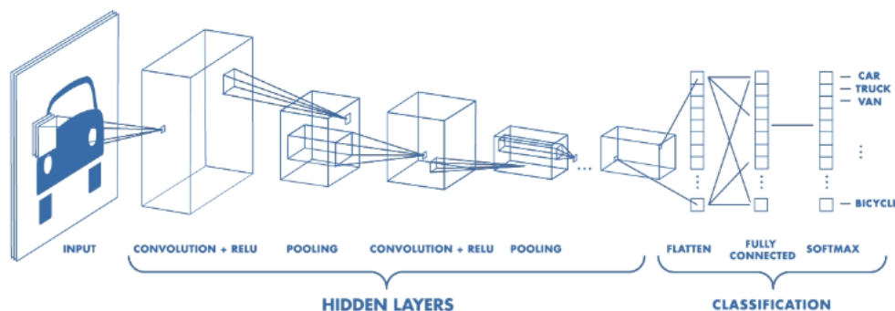
4. ábra. A CNN szerkezete. Az ábra Purwono et al. (2022) [21] cikkéből származik.
