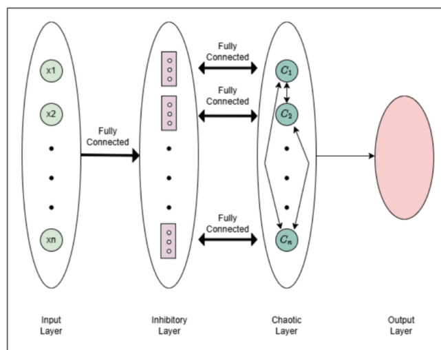
6. ábra. A kaotikus neuron szerkezete Crook & Scheper (2001) [7] alapján. Az ábra Anusree & Pramod (2025) [3] cikkéből származik.
