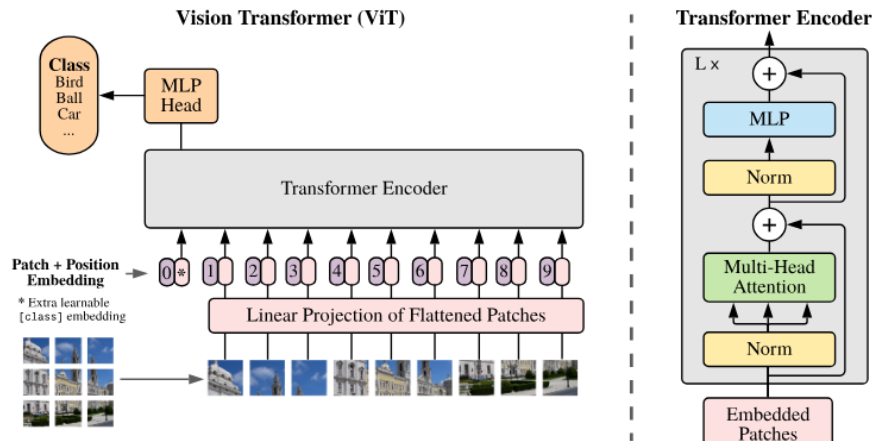
5. ábra. A ViT szerkezete. Az ábra Dosovitskiy et al. (2021) [9] cikkéből származik.
