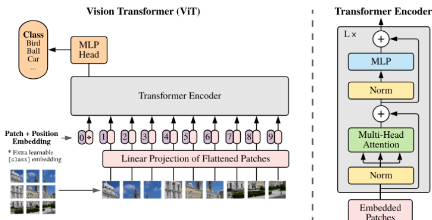
1.5. ábra. A ViT szerkezete. Az ábra Dosovitskiy et al. (2021) [11] cikkéből származik.
