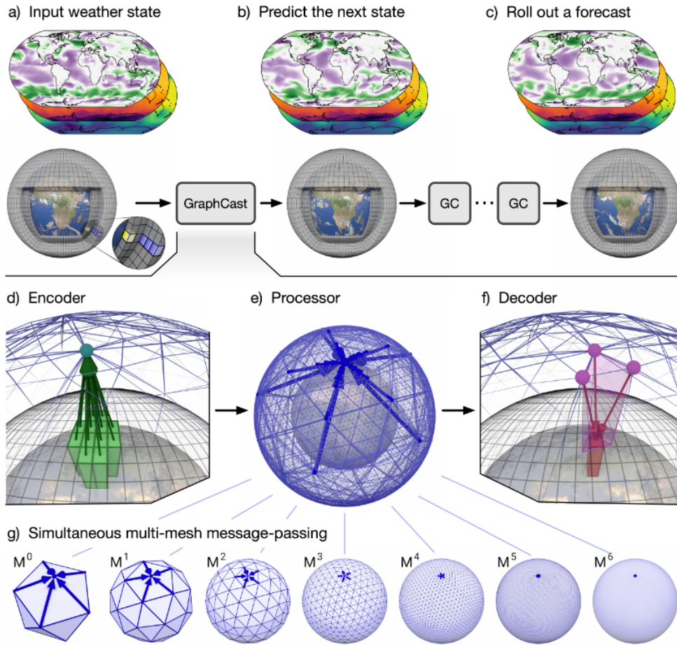
1.8. ábra. A GraphCast modell működése. Az ábra Lam et al. (2023) [18] cikkéből származik.
