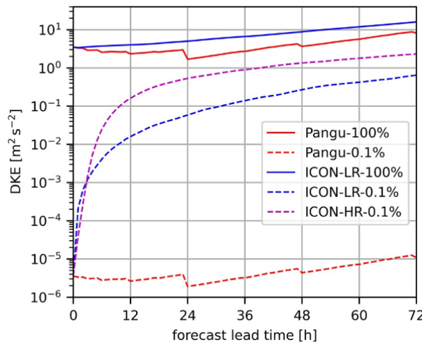
1.10. ábra. Az ICON és Pangu-Weather ( Pangu ) nagy (100%) és kicsi (0.1 %) perturbációkra adott válasza a DKE növekedésén keresztül bemutatva. A HR a nagy felbontást (2.5 km), a LR az alacsony felbontást (20 km) jelent. Az ábra Selz & Craig (2023) [30] cikkéből származik.
