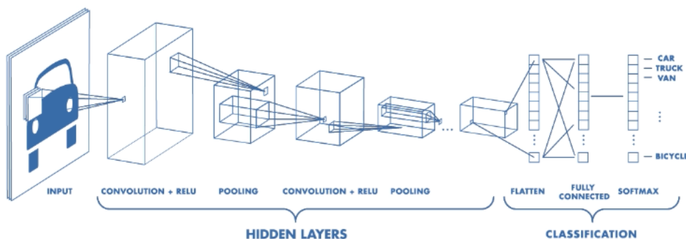
1.4. ábra. A CNN szerkezete. Az ábra Purwono et al. (2022) [27] cikkéből származik.
