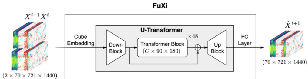
1.9. ábra. A FuXi modell áttekintő szerkezete. Az ábra Chen et al. (2023) [7] cikkéből származik.
