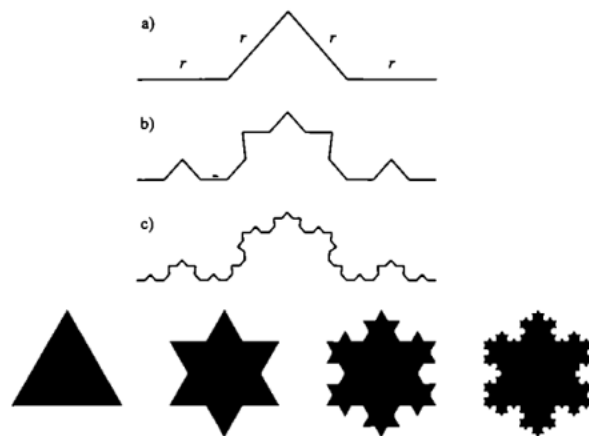
1.11. ábra. A Koch-görbe szerkesztése és fraktálszerkezete. Az ábrák Tél & Gruiz Kaotikus dinamika című tankönyvéből (2002) származnak [34].
