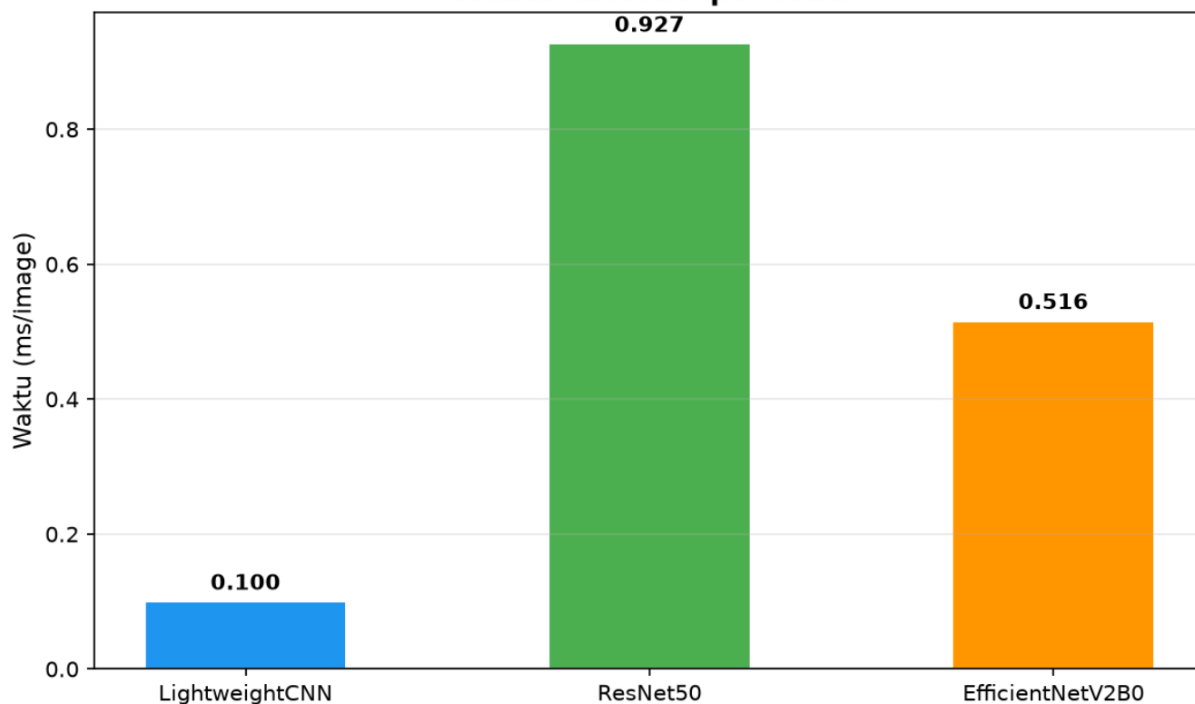
Waktu Inferensi per Citra
