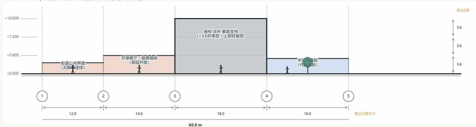
A—A' | 主剖面：街道—首层开放—共享层—驻留层
