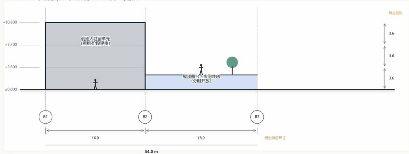
B—B' | 补充剖面：驻留单元—屋顶露台—分时使用
