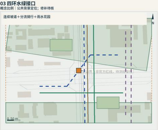
R03-03 | 四环水绿接口
