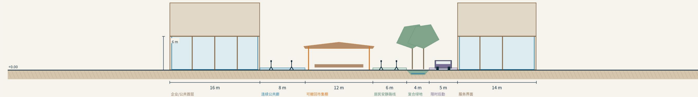
04 A-A 条件性站城-街道-公共首层 | 1:200
