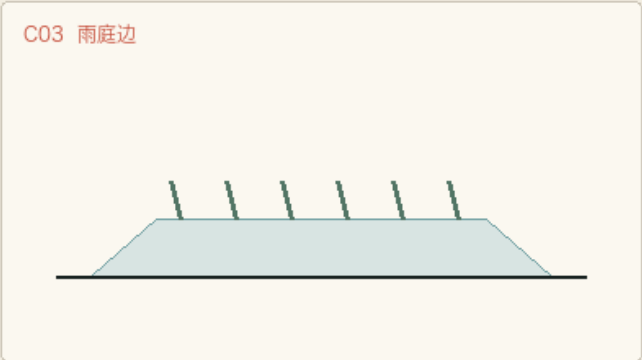
碎石 植草沟 可清淤
