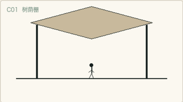
钢柱 木格栅 螺栓连接
