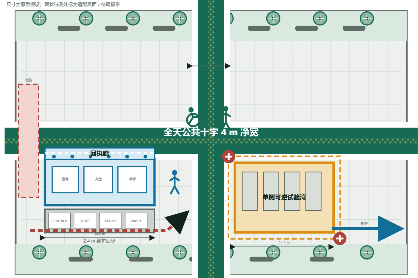
大钟寺·可建造的公共十字 | 1:500 建筑与场地平面
