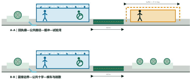
两道 1:200 空间剖面 | 公共基线和插件有清楚的物理边界
