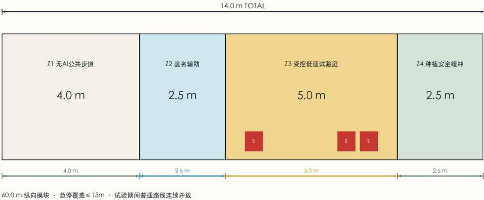
P01 · 尺寸化平面 / DIMENSIONED PLAN · NTS
