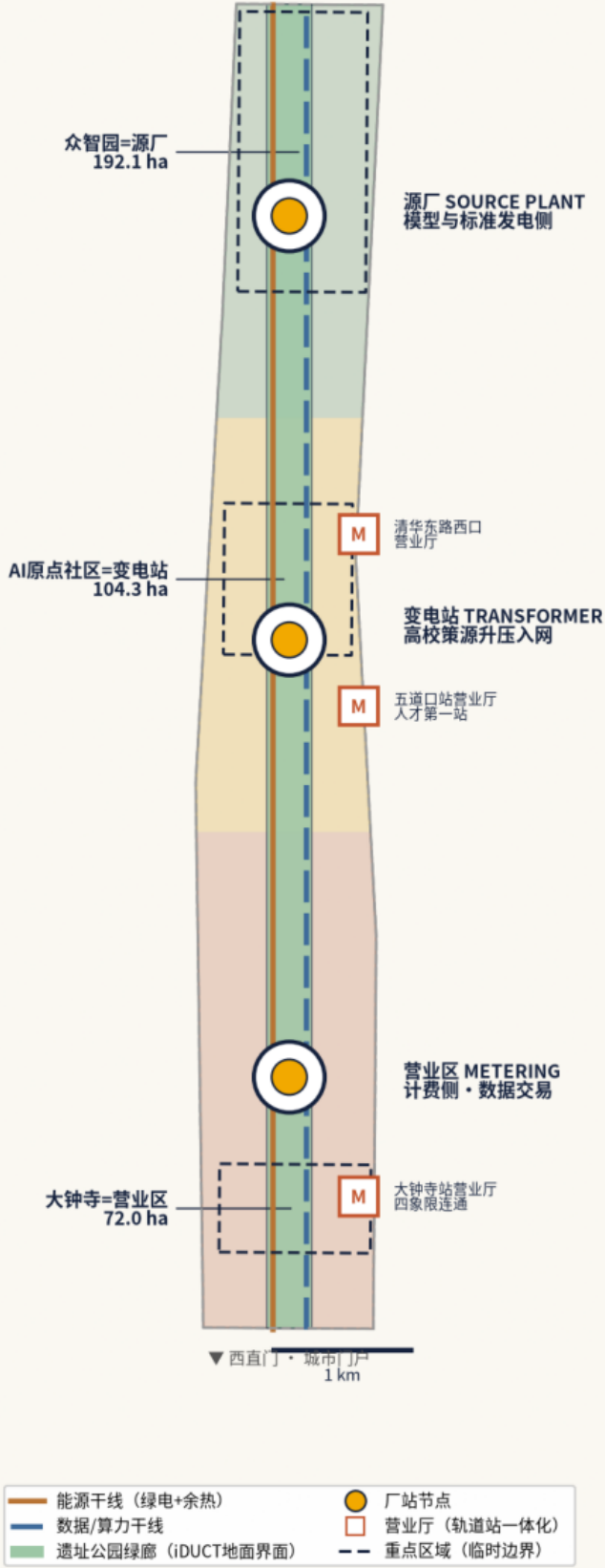
京张通智 JINGZHANG UTILITY · 图1 一沟三厂站总体结构
