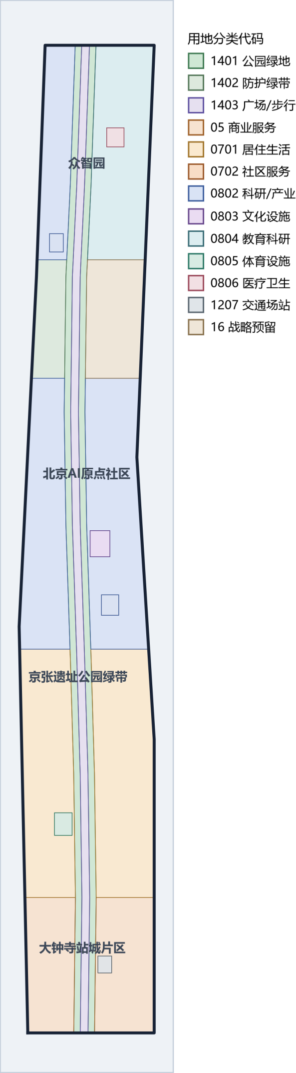
图 2 · 用地结构与功能分区：19 个分区，绿带连续、站城复合、研发聚集。
