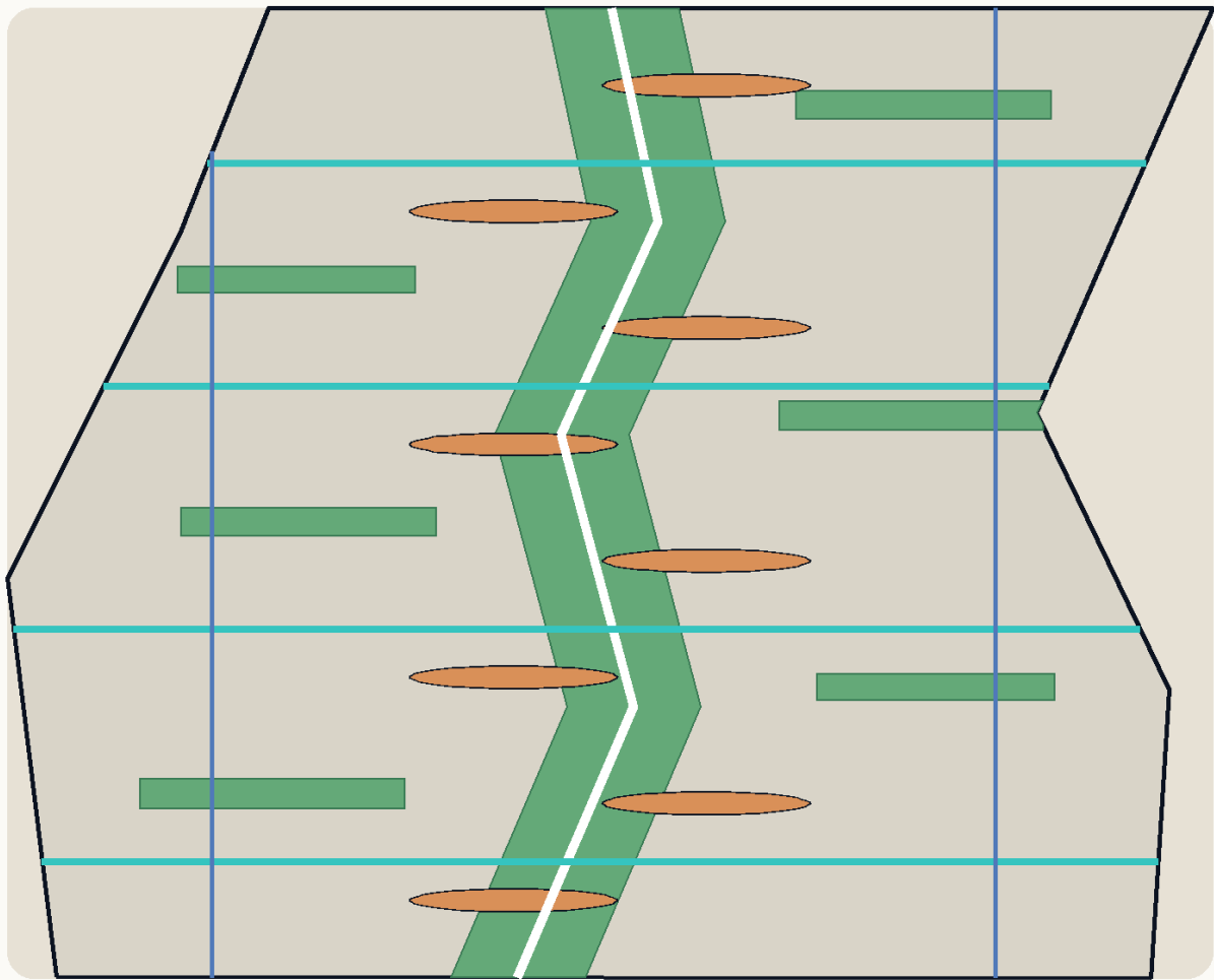
可维护街道剖面
