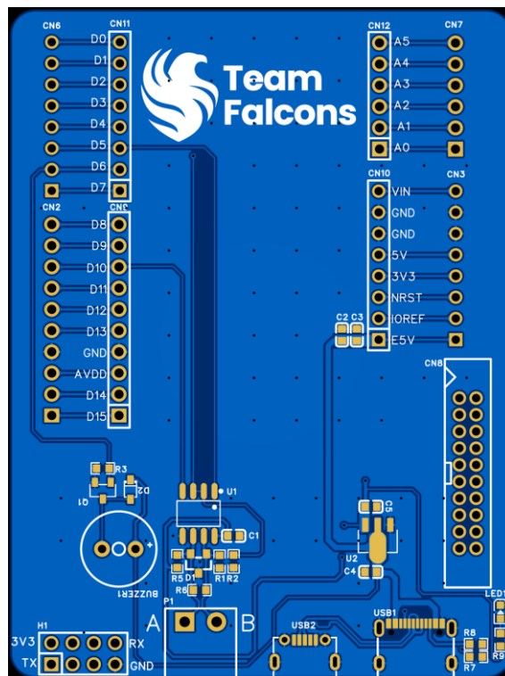
图 14 扩展板 PCB 布局
