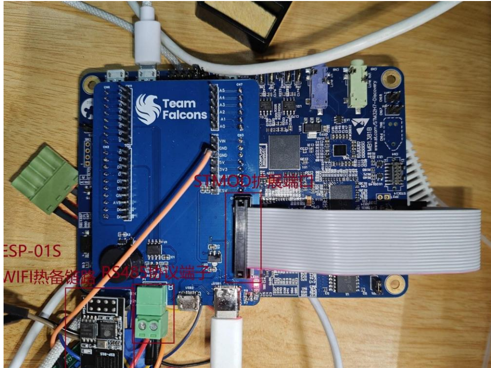
图 12 扩展板与主板的叠插关系
