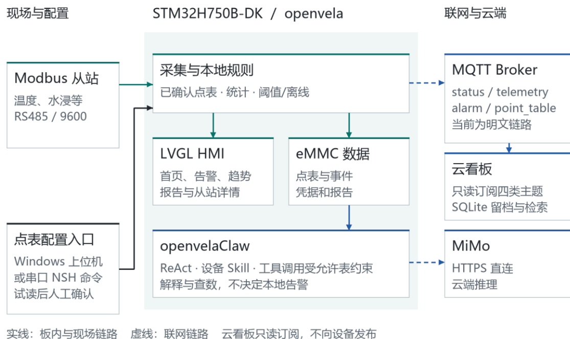
图 2 系统总体架构：现场、板端与云端的职责分工
