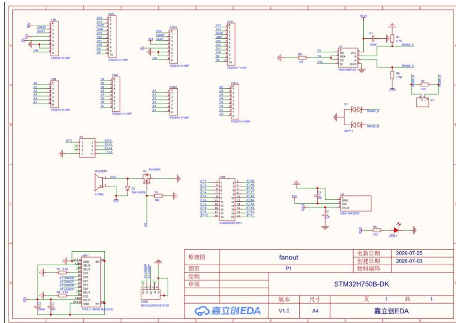
图 13 扩展板原理图：RS485 收发与总线保护、数字量输出与电源
