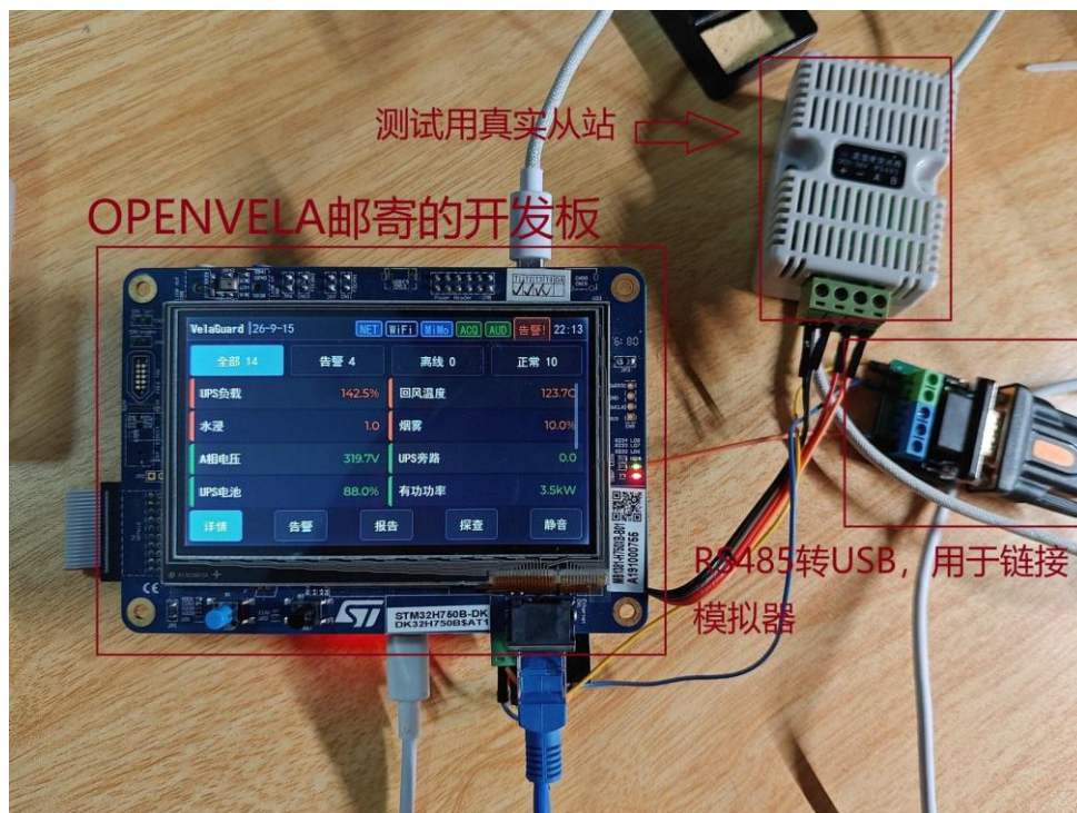
图 3 实物联调拓扑：网关、真实 Modbus 从站与总线模拟器
