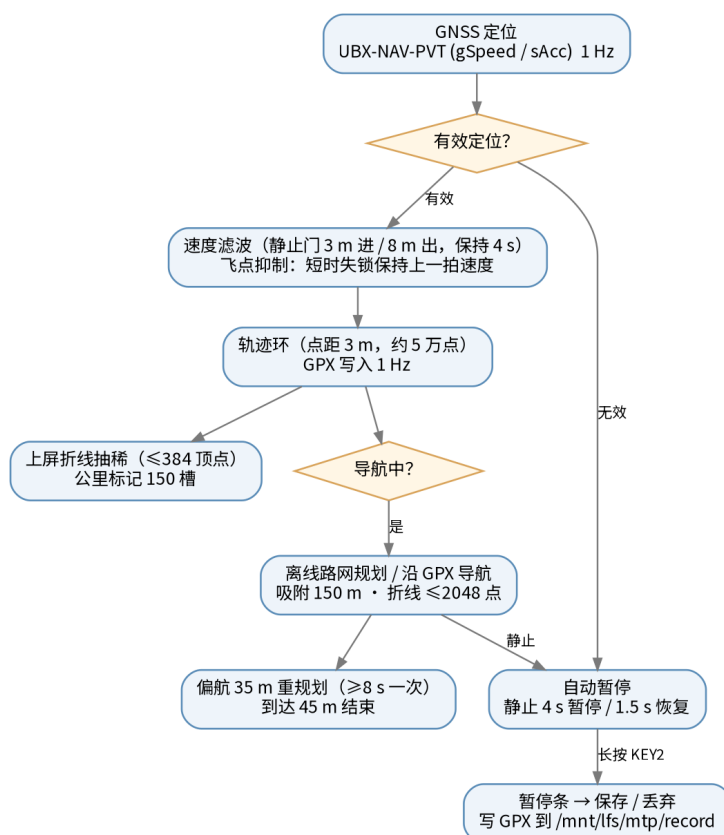
图 3 记录与导航的关键流程
