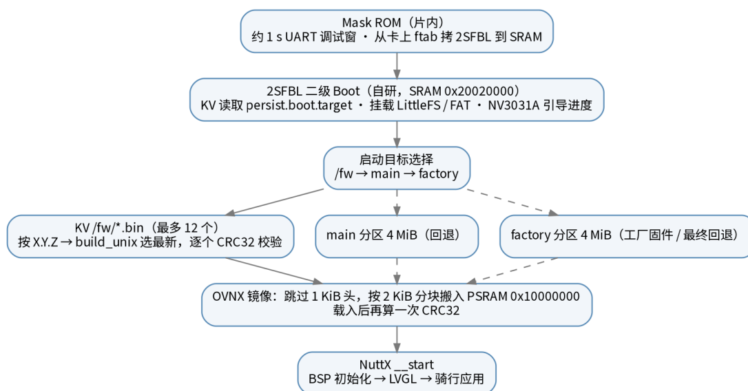
图 2 启动链: Mask ROM → 2SFBL → OVNX → NuttX
