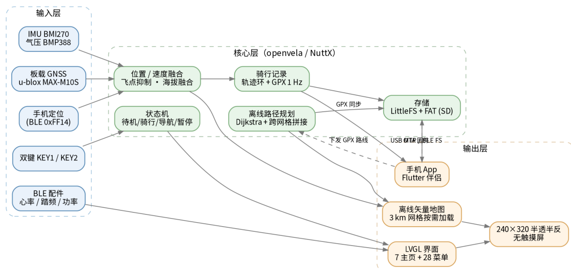
图 1 系统总体架构与数据流
