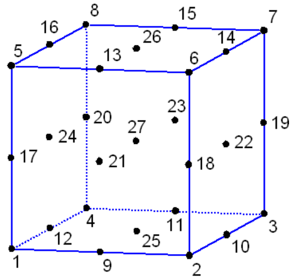
ET_HEX27
