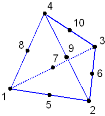
ET_TET10
