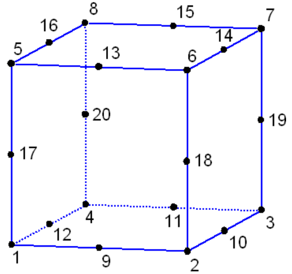
ET_HEX20
