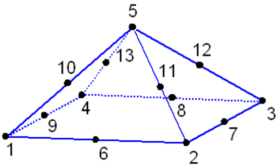
ET_PYRA13
