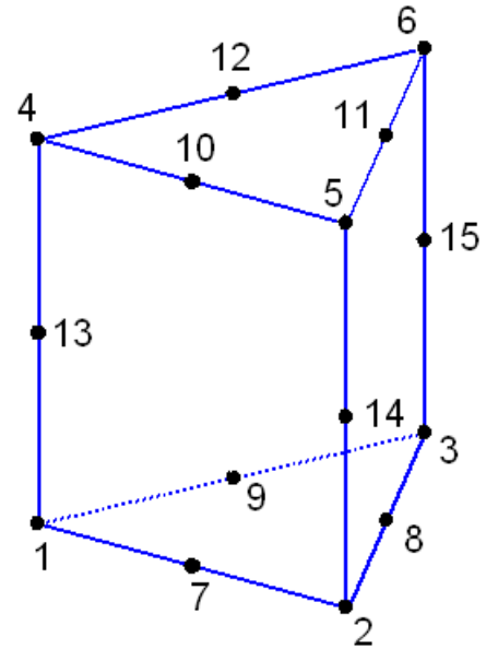
ET_WEDGE15
