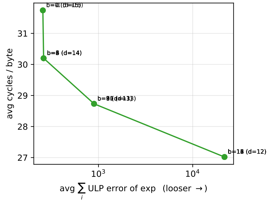
f64
