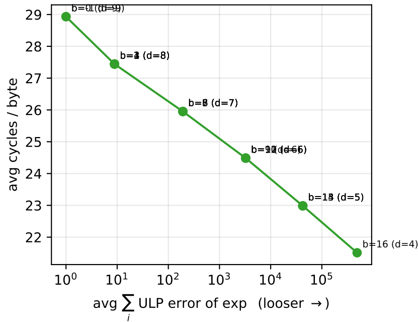
f32
