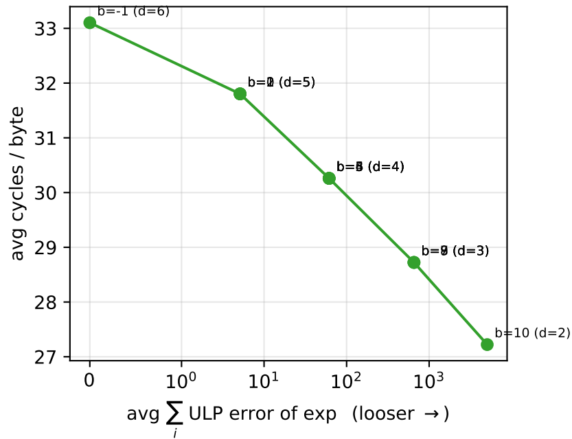
f16
