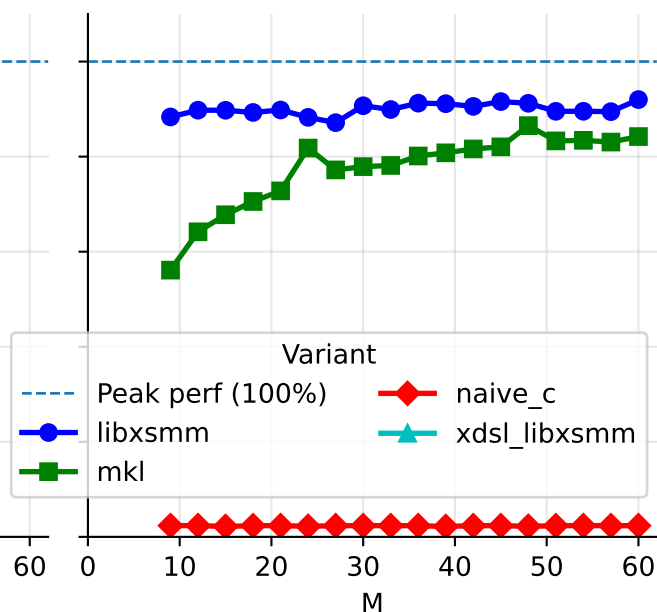
(d) N = K = 64 , f64 , Intel Skylake
