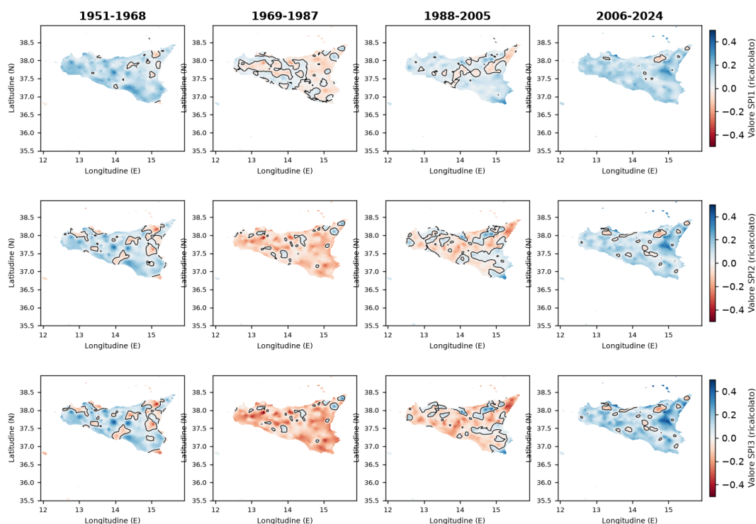
Figura 10: Le mappe della siccità nei quattro periodi (in rosso le zone più secche, in blu le più umide). L'ultima colonna, gli anni più recenti, è in prevalenza blu.
