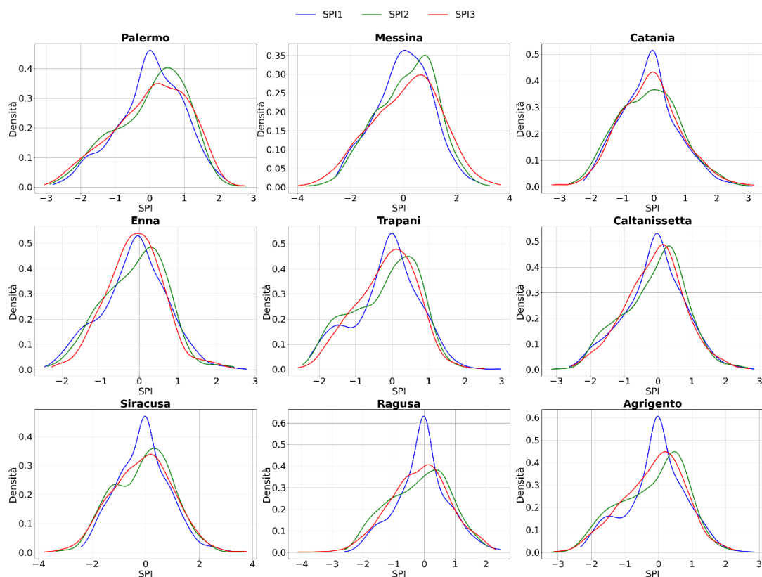
Figura 6: Fig. 9 — dati forniti (originale). Densità SPI per provincia: forme irregolari, talvolta bimodali (es. Trapani, Ragusa, Agrigento).
