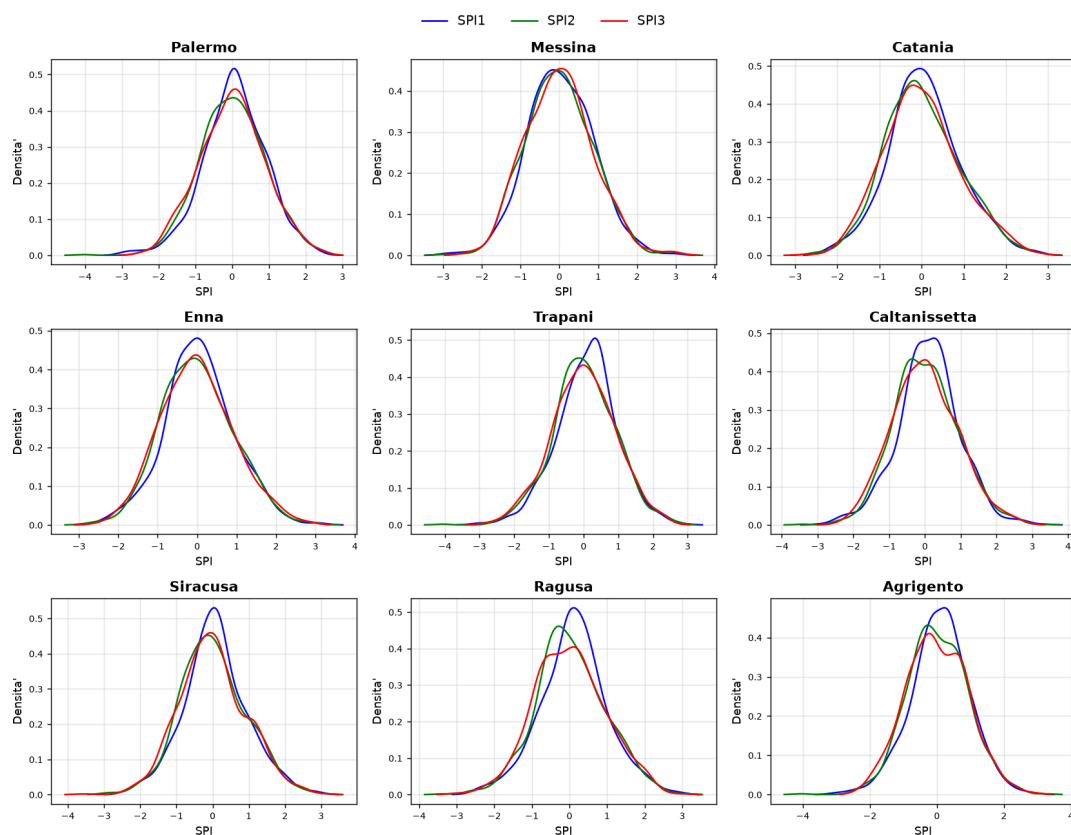
Figura 7: Fig. 9 — dati ricalcolati. Curve regolari e centrate su 0, prossime alla normale standard, come atteso per uno SPI ben definito.
