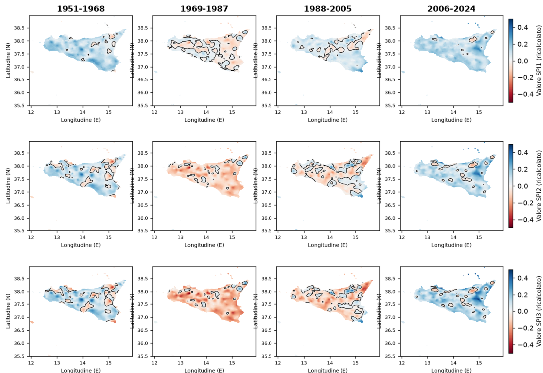
Figura 5: Fig. 8 — dati ricalcolati. Stessa figura con lo SPI standard: il periodo recente (ultima colonna) risulta prevalentemente umido (blu).
