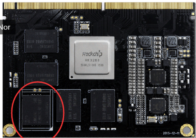
1 EMMC
