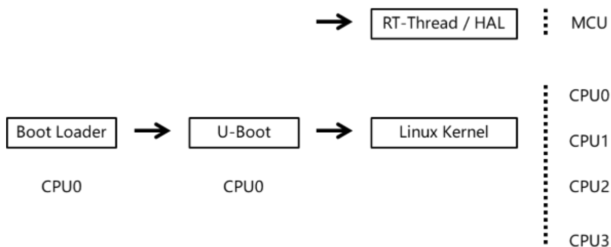
图 5-1-6 kernel + mcu rtt / hal
