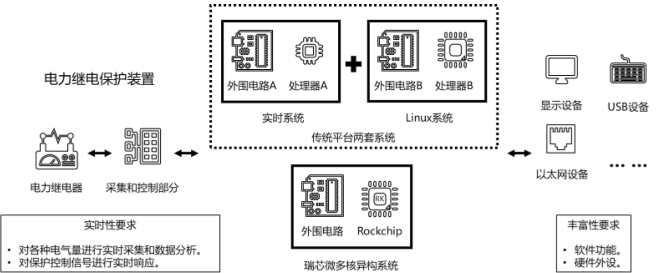
图 3-1-1 AP + AP 案例：电力继电保护装置
