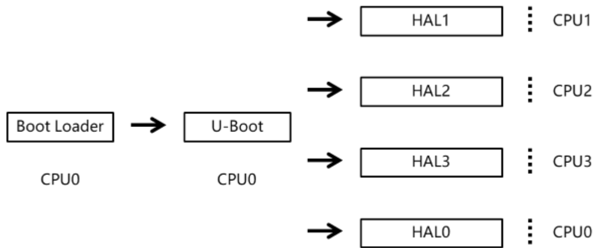
图 5-1-4 hal + hal + hal + hal
