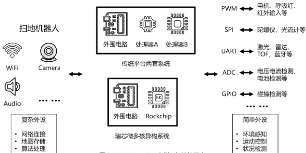
图 3-2-1 AP + MCU 案例：扫地机器人
