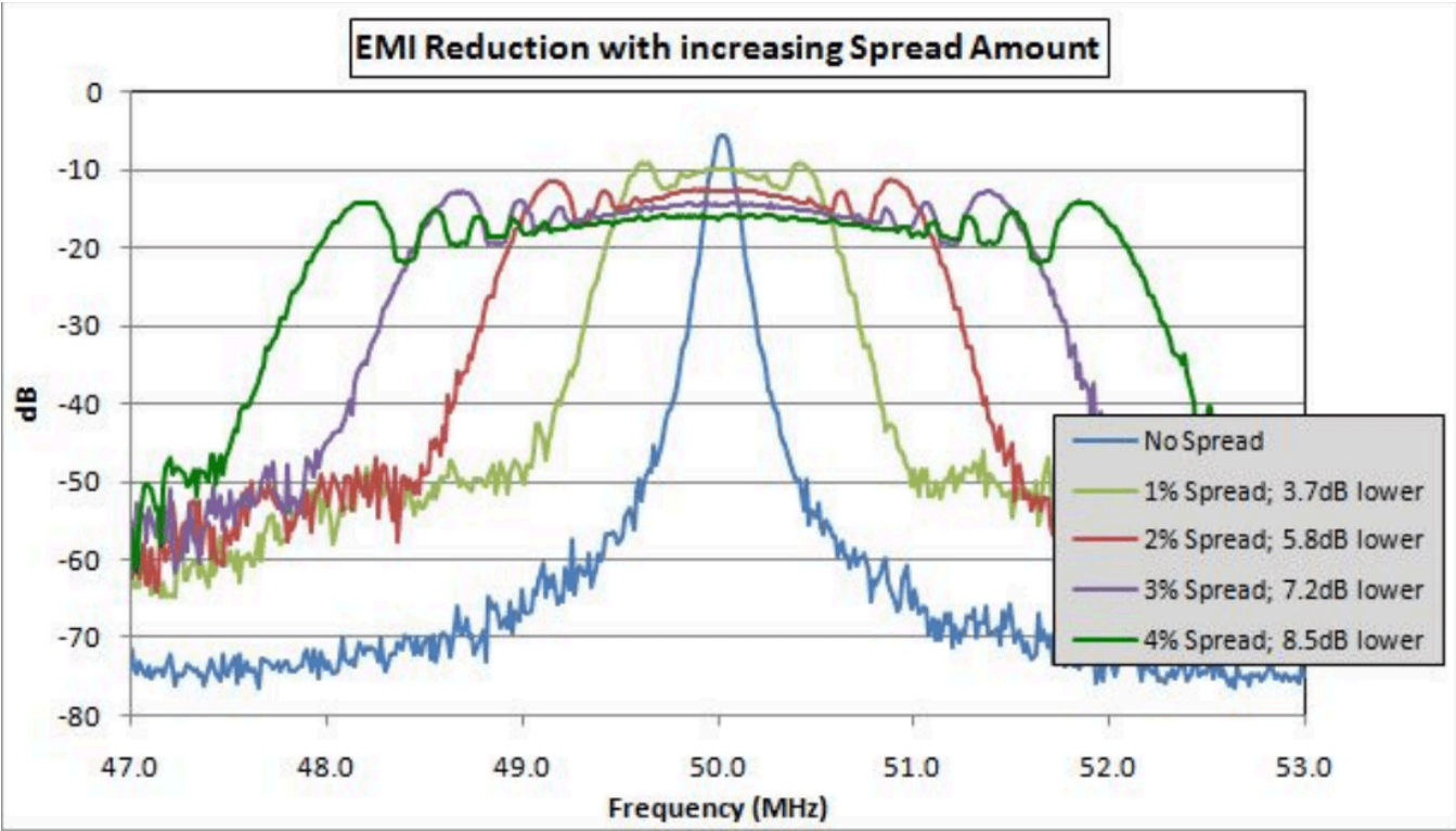
图2示不同调制深度下，EMI峰值的对比。
