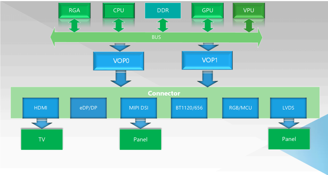
VOP 1.0 显示子系统架构
