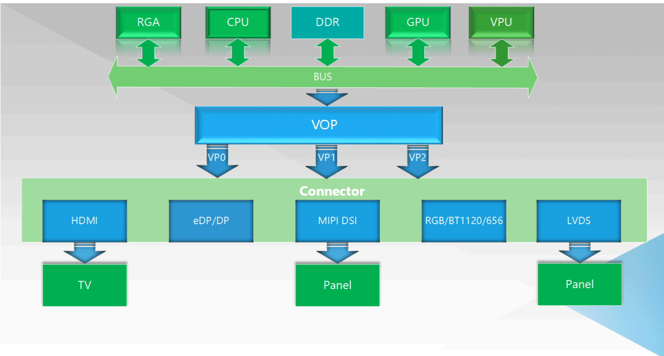
VOP 2.0 显示子系统架构
