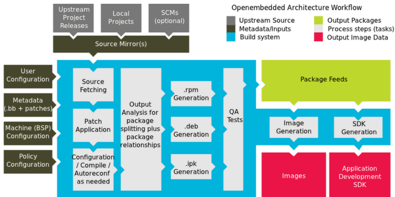
图2-1 Yocto编译框图
