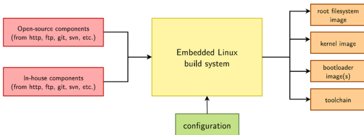
图1-1 Buildroot编译框图
