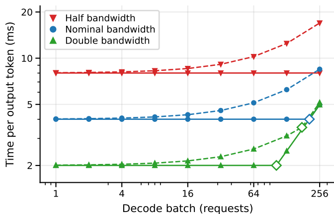
(d) 70B-class dense, TP8 H200 bandwidth sweep
