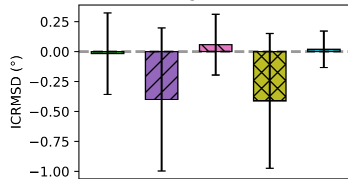
Angle RMSD
