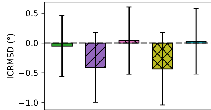
Angle RMSD
