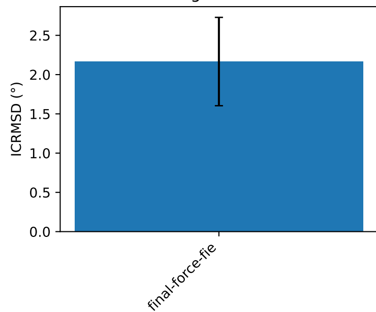
Angle RMSD
