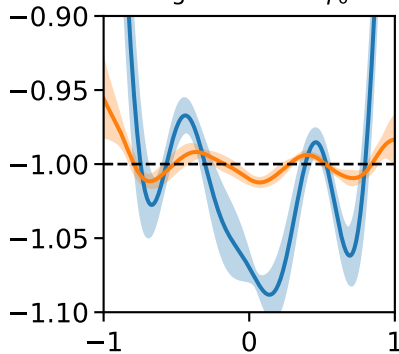
Eigenfunction \psi_0
