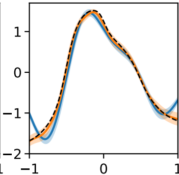
Eigenfunction \psi_2
